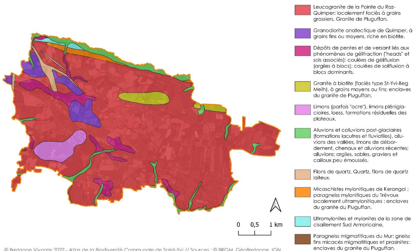
Figure 4 : géologie de Saint-Yvi.
